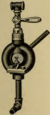
FIG. 16.—THE SIPHON.
